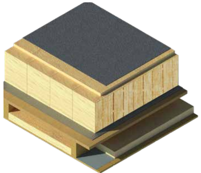
Fig. 17: Principkonstruktion på parallelltak
