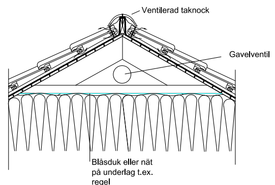
2.16 Blåsduk som mothåll.
