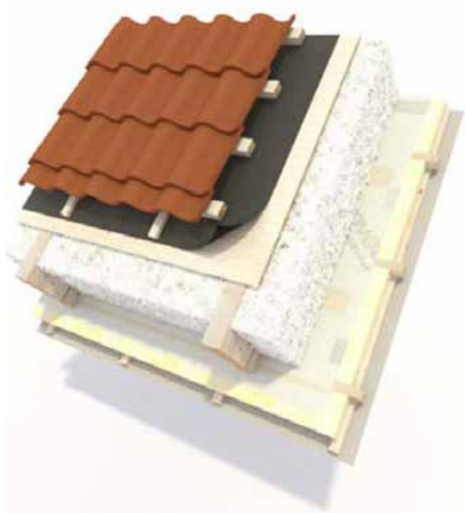
Kompakt tak med ISOVER InsulSafe.
