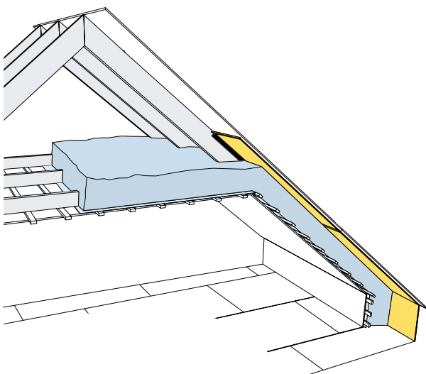
Vindavledare snedtak
