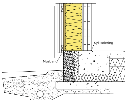
Grunddetalj alt. 2
