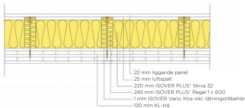
Horizontalsnitt, ISOVER PLUS+ på massivträ
