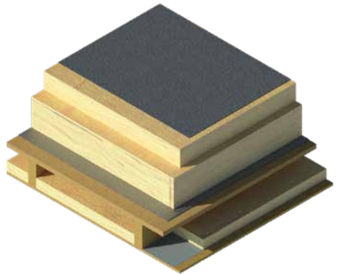
Fig. 20: Flerskiktsslösning på parallelltak med ISOVER ROBUST Takskira
