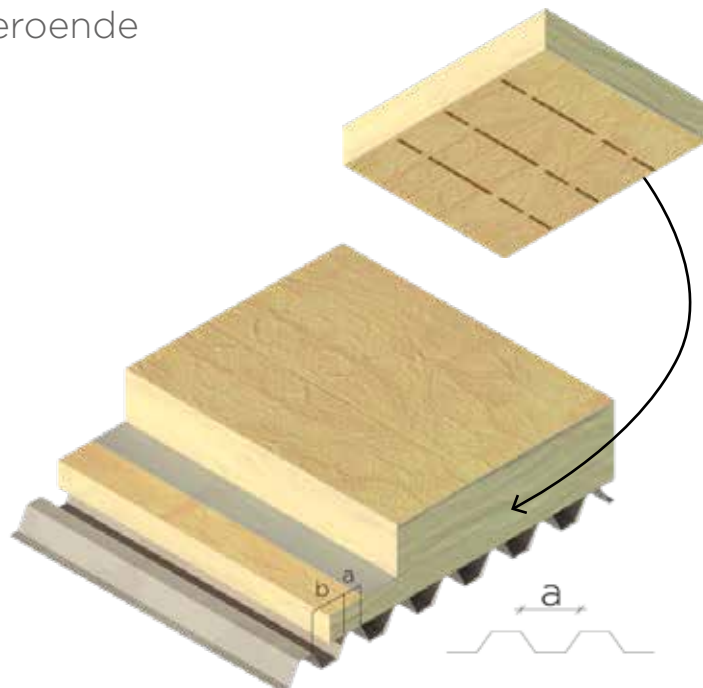
Fig. 7: ISOVER ROBUST skivskarv oberoende av profiltopp
