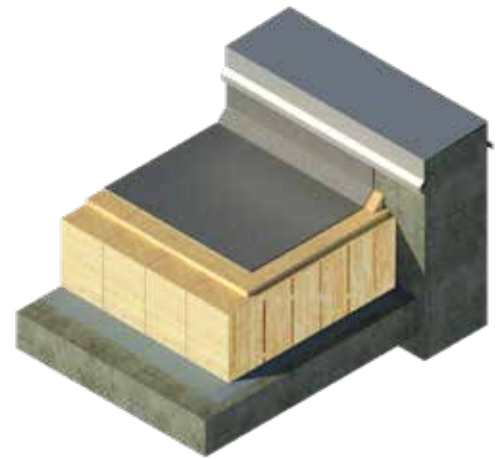
Fig. 4: ISOVER ROBUST Lamell på underlag av betong
